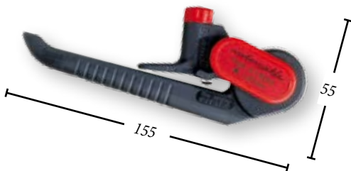
Dụng cụ lột vỏ cáp AMS - AV6221
